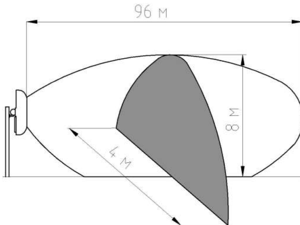
Рисунок 8.1 Зона обнаружения извещателя при установке на участке периметра
