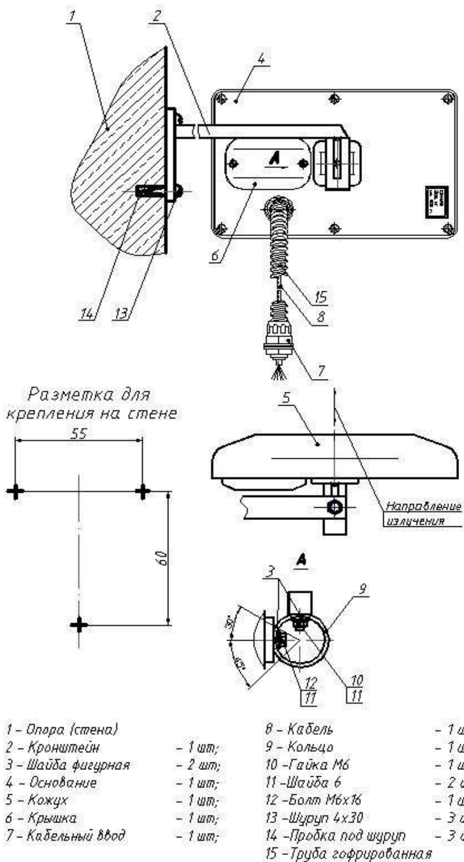
Рисунок 6.2 Установка извещателя на стене с помощью кронштейна 120 мм.
