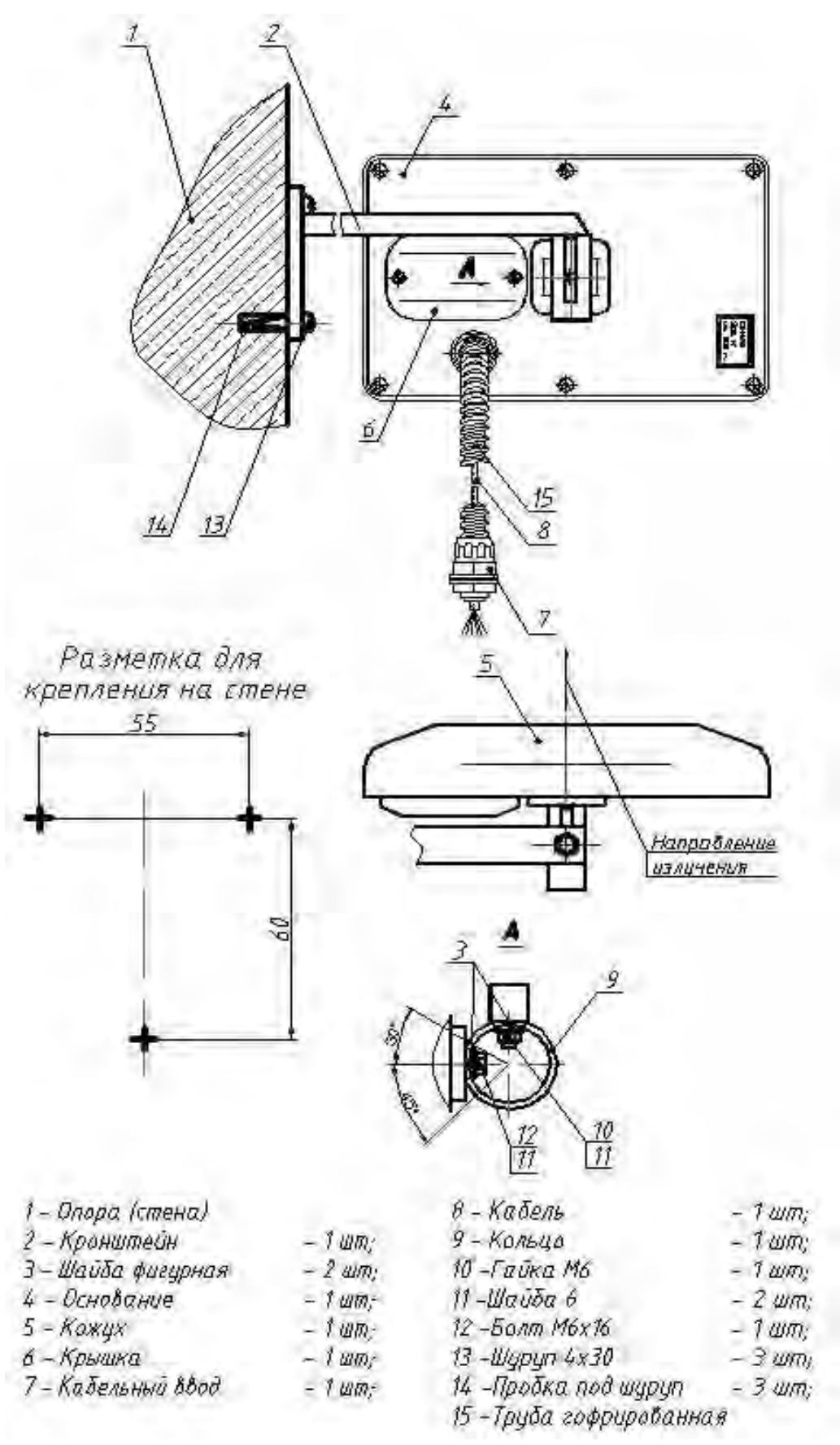
Рисунок 6.2 Установка извещателя на стене (вариант исполнения - штора)
