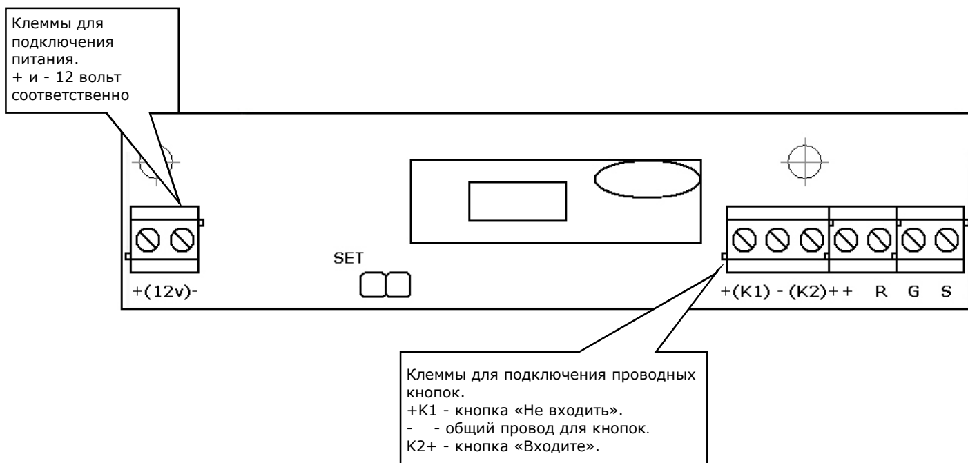
Рисунок 6.1. Печатная плата на задней стороне корпуса светозвукового табло
