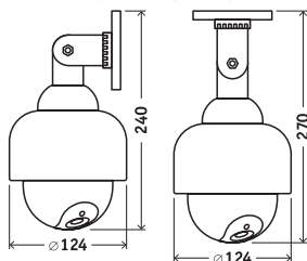
Габаритные размеры
