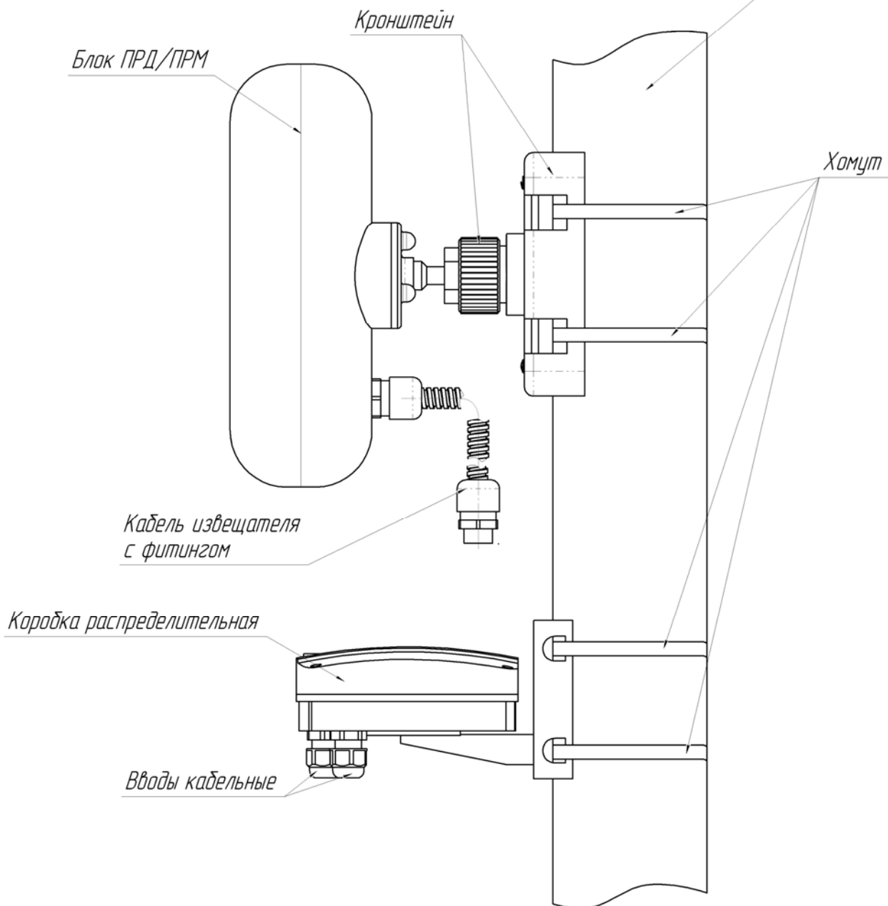
Рисунок 1.2 – Внешний вид блока ПРМ/ПРД «ТАНТАЛ-200-01» и КР на опоре
