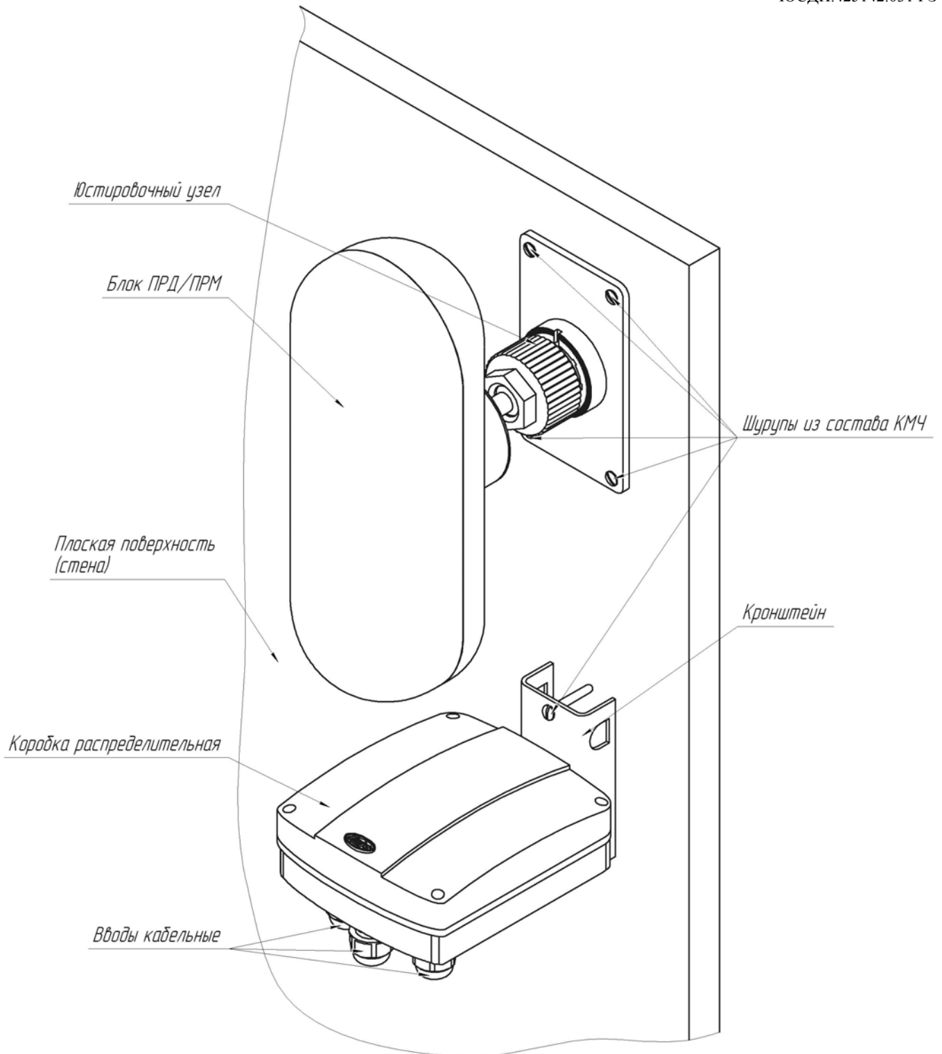
Рисунок 1.3 – Внешний вид блоков ПРМ /ПРД «ТАНТАЛ-200-01» и КР на плоской поверхности (стене)
