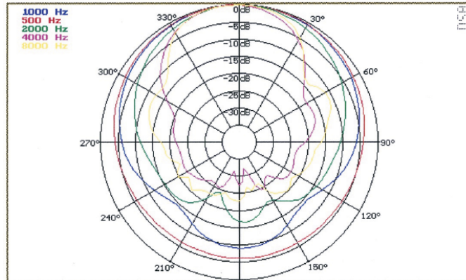
Частотная характеристика и характеристика направленности громкоговорителя
