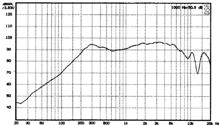
Частотная характеристика и характеристика направленности громкоговорителя
