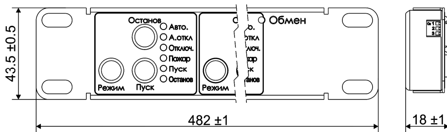
Рисунок 8 – Габаритные размеры «Тунгус ПИ»
