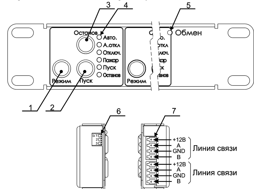
Рисунок 9 – Органы управления и разъёмы «Тунгус ПИ»
