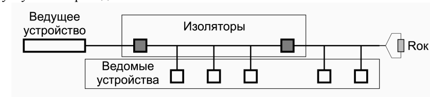
Рисунок 17 – Топология «луч»
