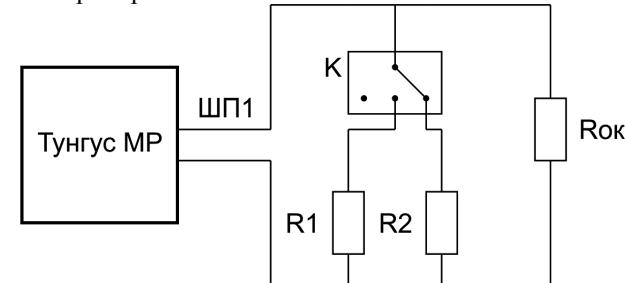
Рисунок 11 – Подключение УВОА к модулю расширения\
