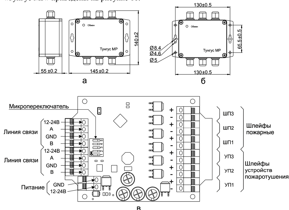
Рисунок 10 – Модуль расширения «Тунгус МР»
