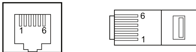
Рисунок 7 – Гнездо и штекер УП1 и УП2
