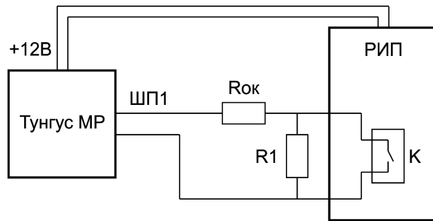
Рисунок 12 – Подключение РИП к модулю расширения
