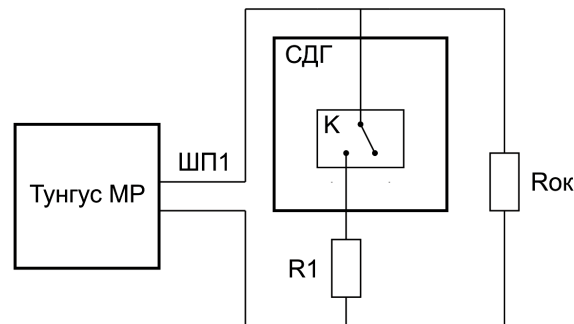
Рисунок 13 – Подключение СДГ к модулю расширения
