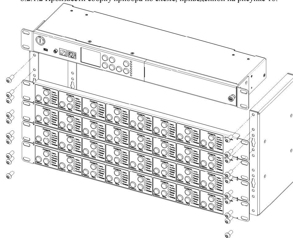
Рисунок 16 – Сборка прибора
