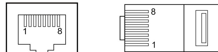
Рисунок 6 – Гнездо и штекер ШП
