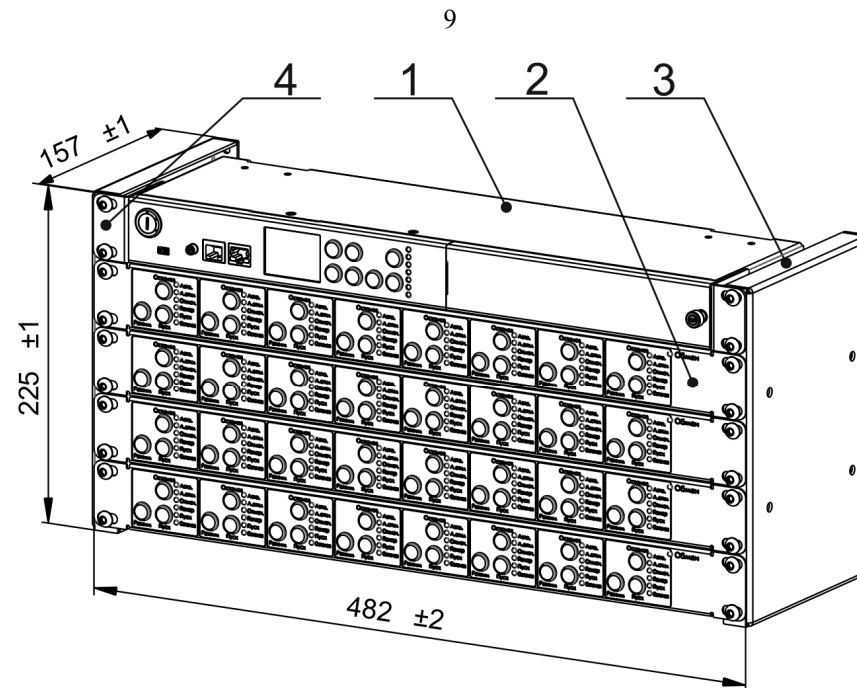
Рисунок 1 – Внешний вид ППКОПиУ
