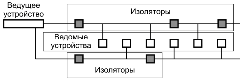
Рисунок 18 – Топология «кольцо»
