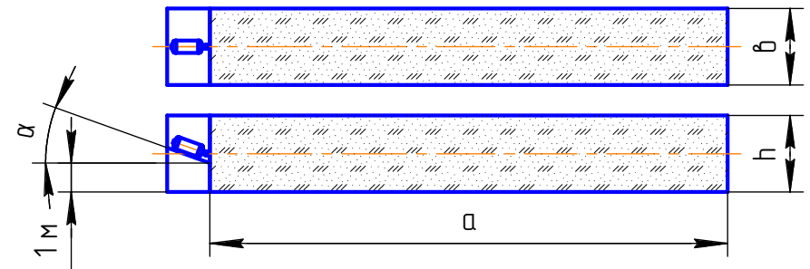
Рисунок 2 - Изображение области, в которой достигается тушение пожара класса А
