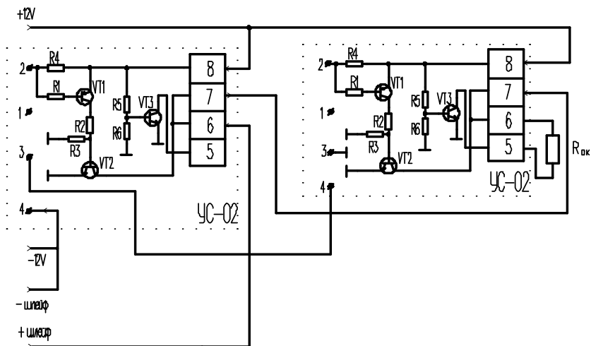
Схема подключения датчиков ИП 212-45 к четырехпроводным концентраторам (с использованием УС-02)
