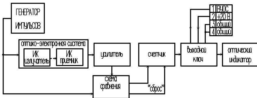
Структурная схема пожарного извещателя ИП 212-45
