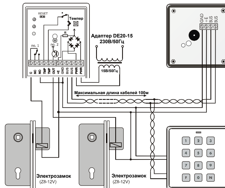
Пример системы для управления двумя дверными электрозамками.
