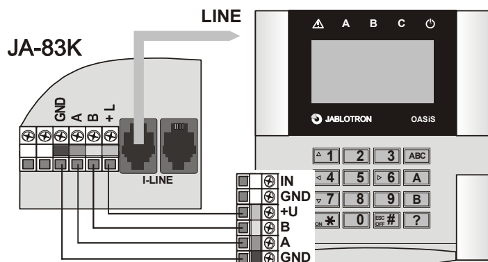
рис. 1 соединение пульта управления с централью
