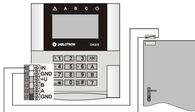
рис. 2 подключение детектора открытия дверей
