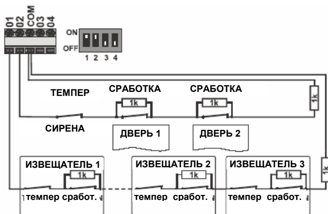
Не более 5 извещателей в шлейфе
