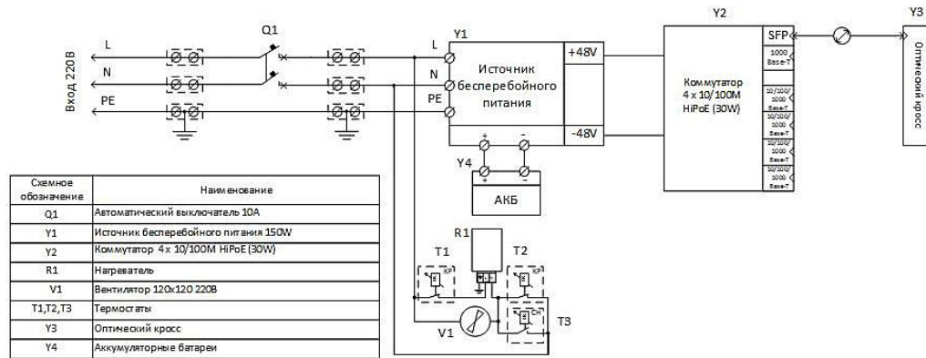
Рис. 1. Электрическая схема Узла доступа NSBox-140-R
