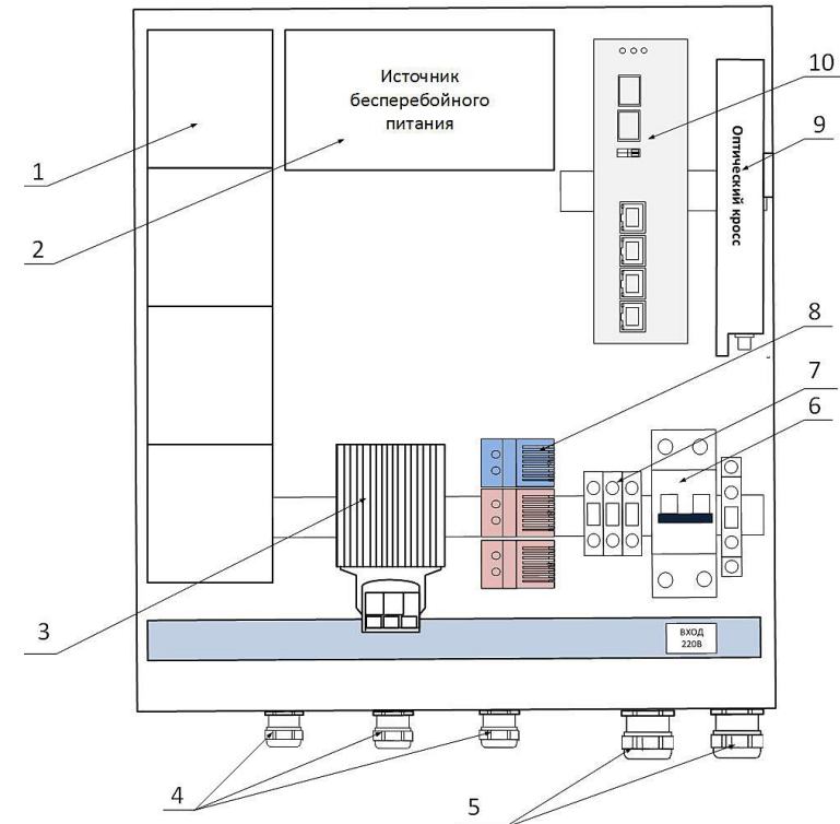
Рис. 2. Базовая комплектация Узла доступа NSBox-140-R*
