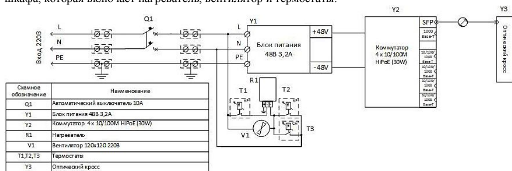
Рис. 1. Электрическая схема Узла доступа NSBox-140
