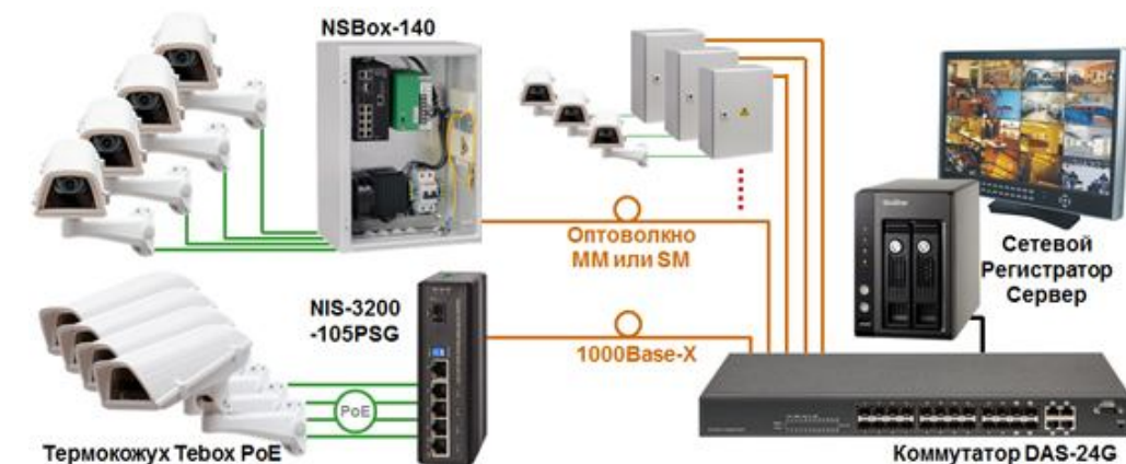
Рис. 1. Электрическая схема Узла доступа NSBox-140
