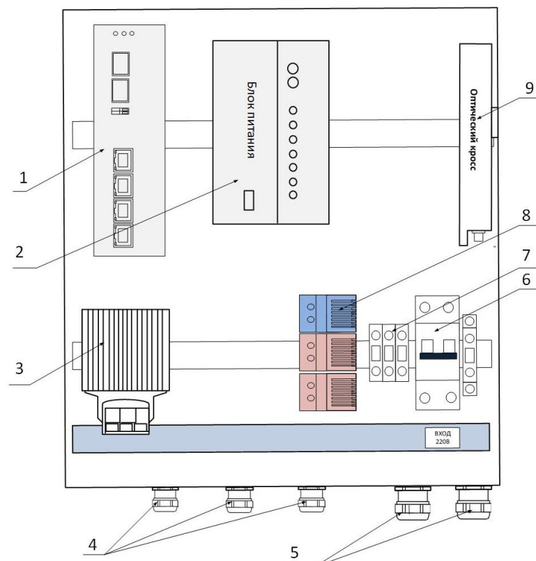
Рис. 2. Базовая комплектация Узла доступа NSBox-140*
