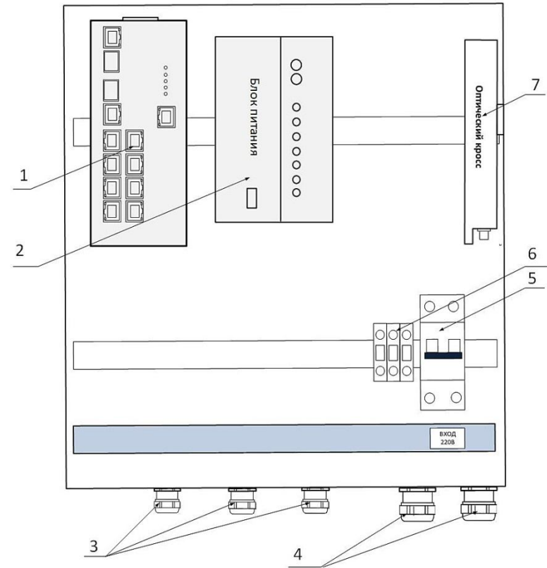
Рис. 2. Базовая комплектация Узла доступа NSBox-180-Н*
