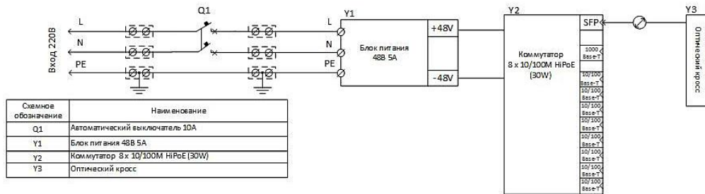
Рис. 1. Электрическая схема Узла доступа NSBox-180-Н
