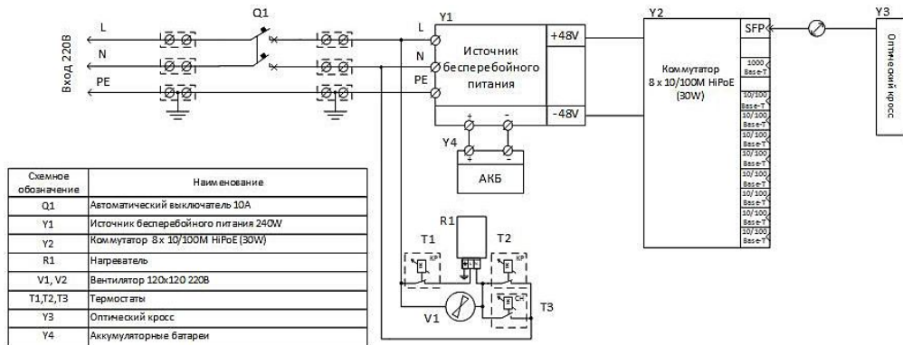
Рис. 1. Электрическая схема Узла доступа NSBox-180-R
