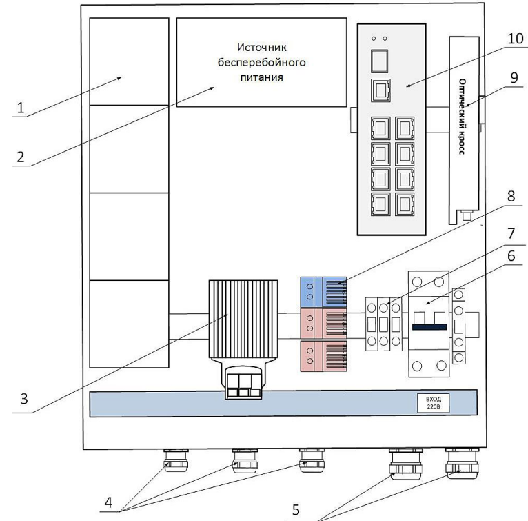
Рис. 2. Базовая комплектация Узла доступа NSBox-180-R*
