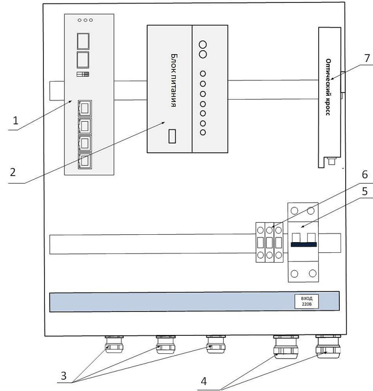
Рис. 2. Базовая комплектация Узла доступа NSBox-243-H*
