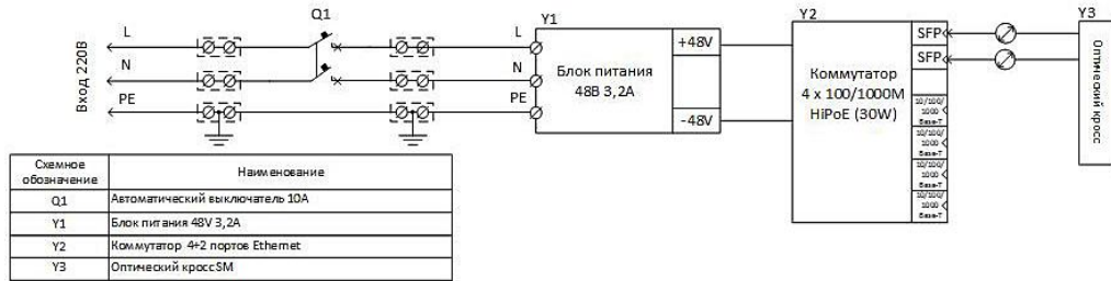
Рис. 1. Электрическая схема Узла доступа NSBox-243-H
