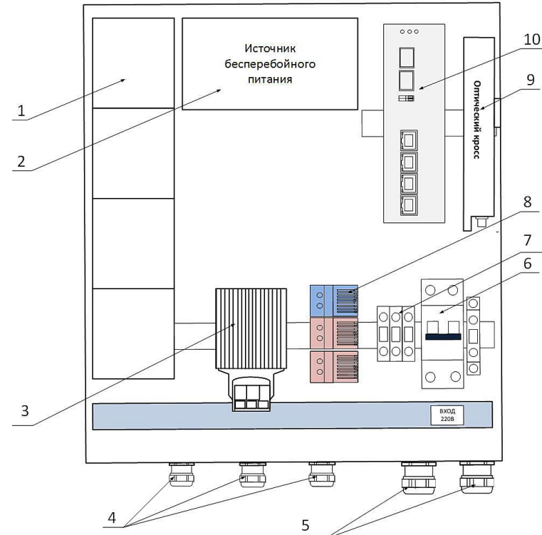
Рис. 2. Базовая комплектация Узла доступа NSBox-243-R*
