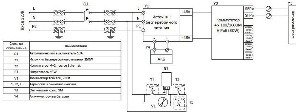
Рис. 1. Электрическая схема Узла доступа NSBox-243-R
