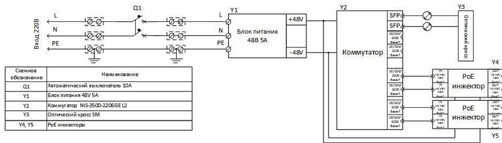
Рис. 1. Электрическая схема Узла доступа NSBox-264-H
