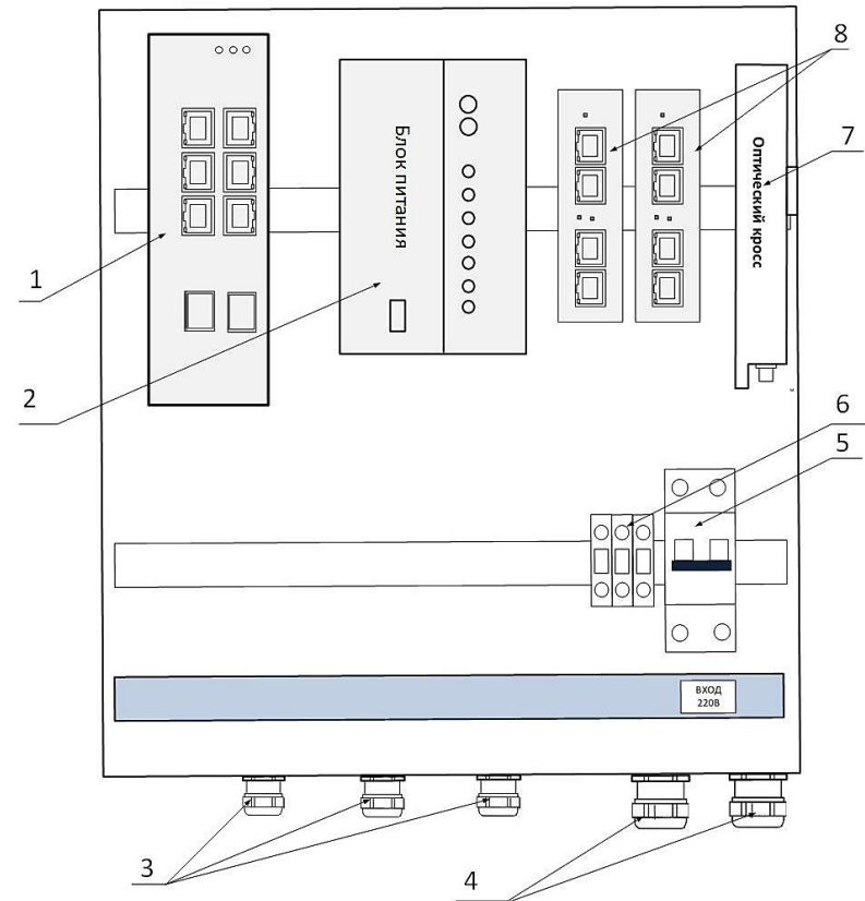
Рис. 2. Базовая комплектация Узла доступа NSBox-264-H*
