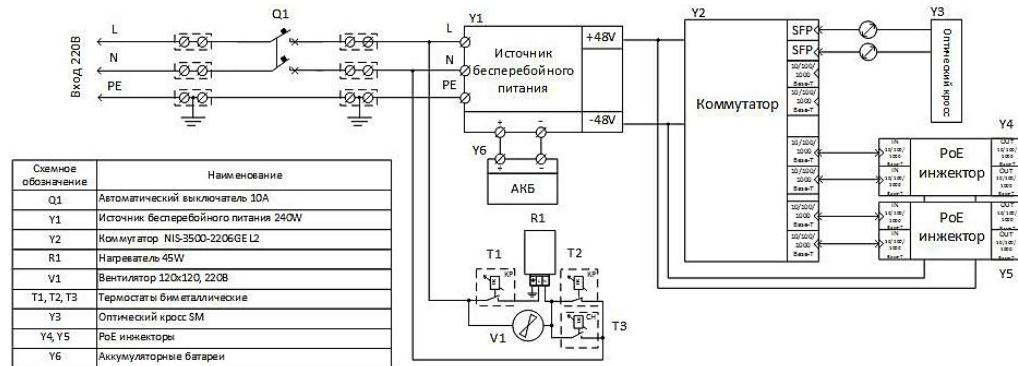
Рис. 1. Электрическая схема Узла доступа NSBox-264-R
