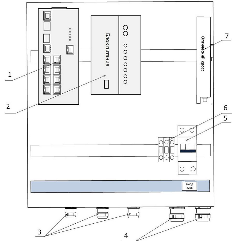
Рис. 2. Базовая комплектация Узла доступа NSBox-280-H*
