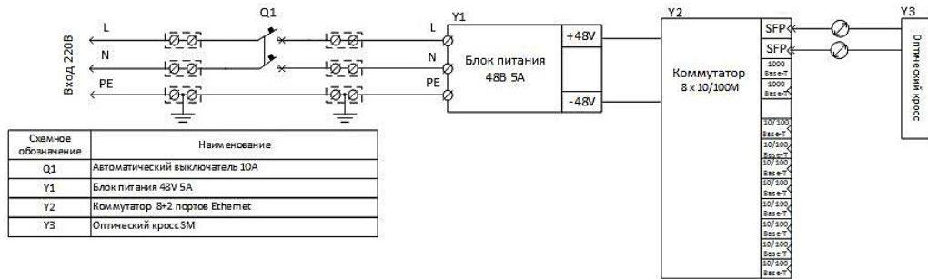
Рис. 1. Электрическая схема Узла доступа NSBox-280-H
