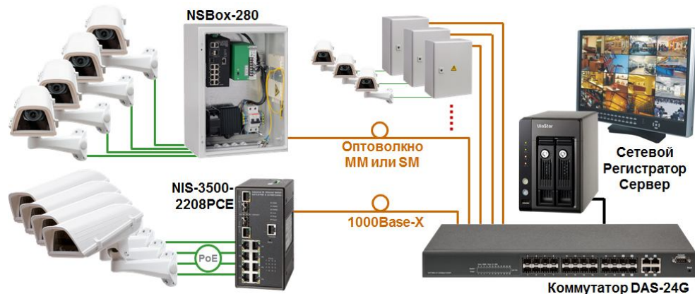
Рис. 1. Электрическая схема Узла доступа NSBox-280-H
