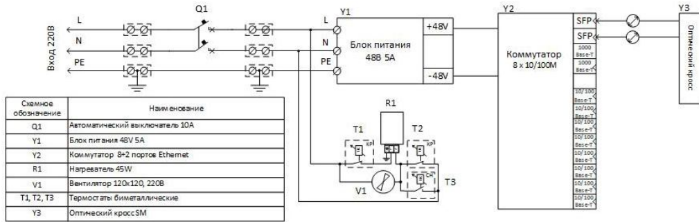
Рис. 1. Электрическая схема Узла доступа NSBox-280
