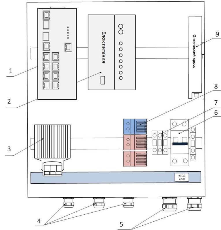
Рис. 2. Базовая комплектация Узла доступа NSBox – 280*
