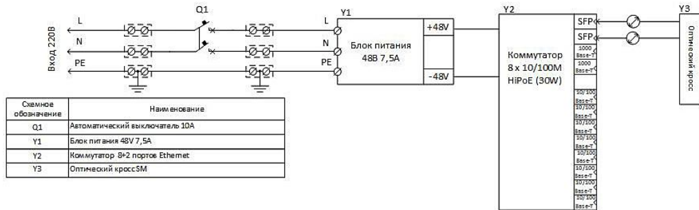
Рис. 1. Электрическая схема Узла доступа NSBox-284-H
