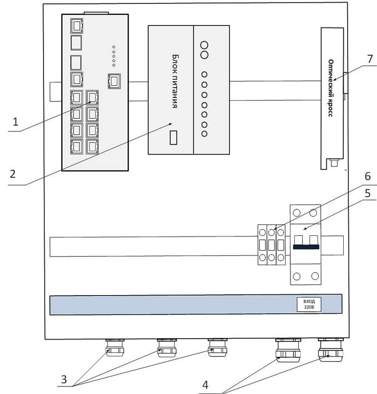
Рис. 2. Базовая комплектация Узла доступа NSBox-284-H*
