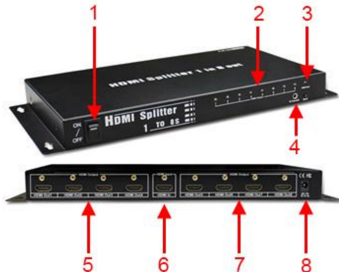
Рис.2 Элементы разветвителя D-Hi108/cascad
