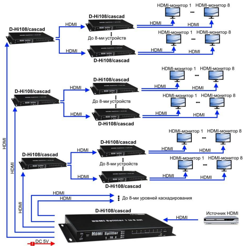
Рис. 3 Схема подключения разветвителя D-Hi108/cascad
