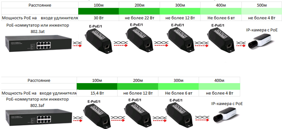
Рис.3 Зависимость передаваемой мощности PoE от расстояния
