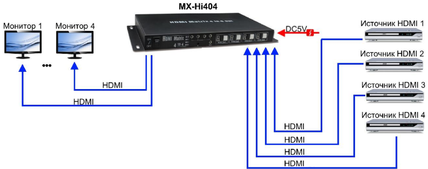
Рис. 3 Схема подключения устройства MX-Hi404
