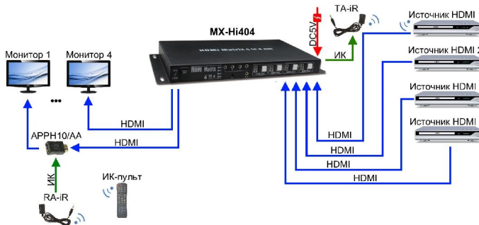
Рис. 4 Схема передачи ИК сигналов коммутатором MX-Hi404
