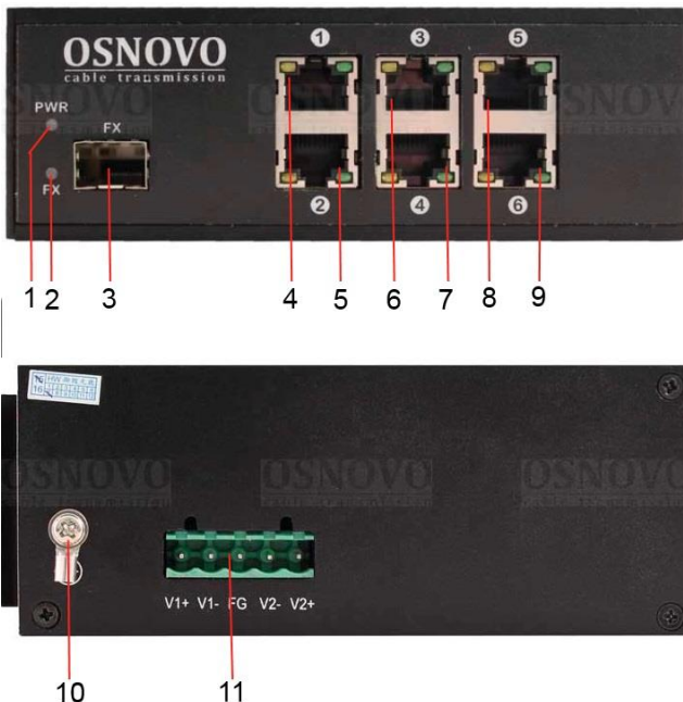
Рис. 3 Разъемы и индикаторы коммутатора SW-40501/IC
