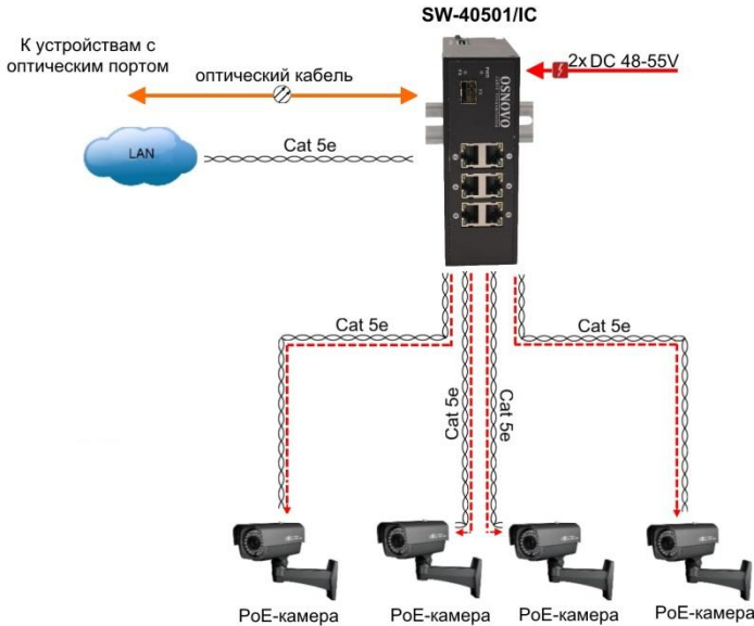
Рис.4 Типовая схема подключения коммутатора SW-40501/IC
