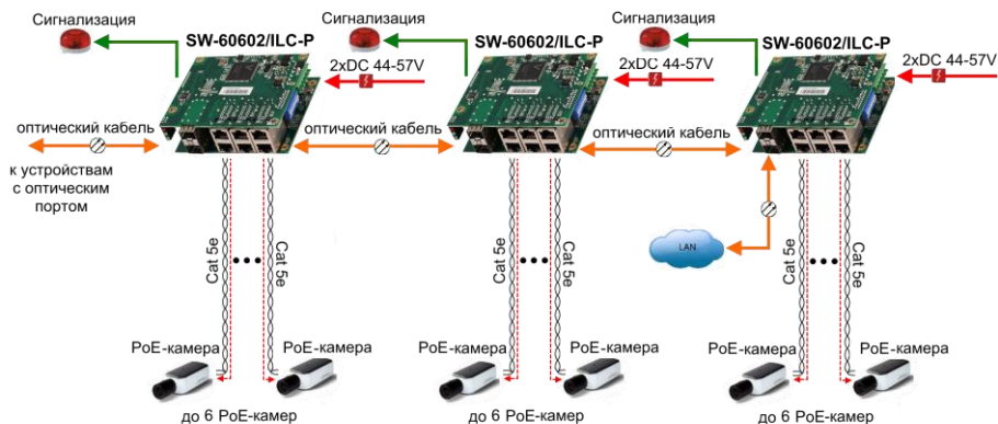
Рис.4 Типовая схема подключения коммутатора SW-60602/ILC-P
