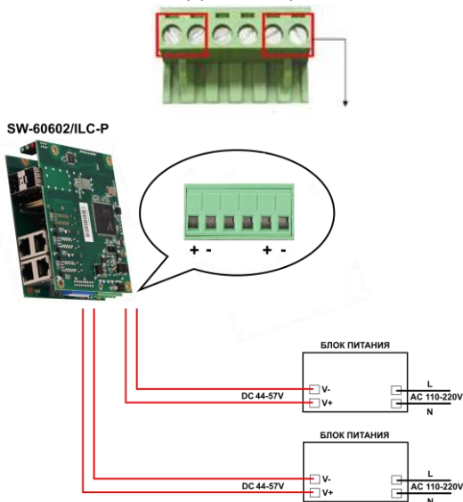
Рис.5 Схема подключения блоков питания к клеммной колодке коммутатора SW-60602/ILC-P.
