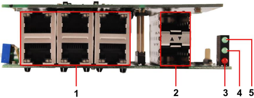
Рис. 2 Коммутатор SW-60602/ILC-P, разъемы, кнопки и индикаторы, вид спереди
