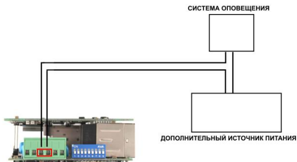
Рис.6 Схема подключения системы оповещения к коммутатору SW-60602/ILC-P.
