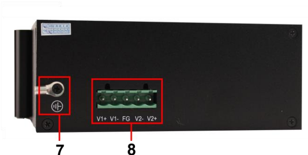
Рис. 3 Разъемы, кнопки и индикаторы коммутатора SW-8062/IC
