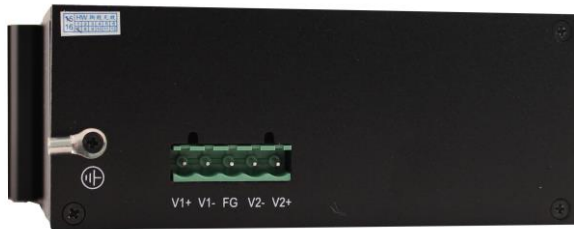
Рис.2 Коммутатор SW-8062/IC, вид спереди/сбоку
