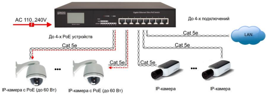
Рис.7 Типовая схема подключения коммутатора SW-8080/THE
