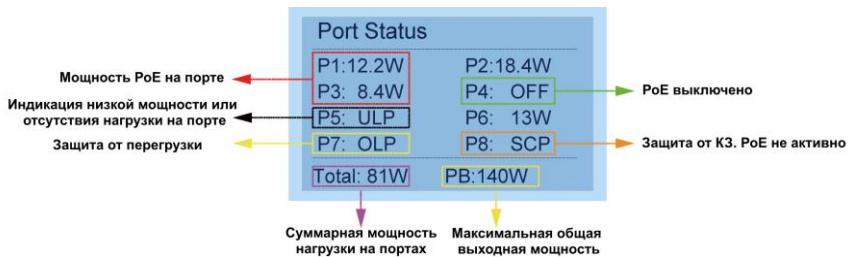
Рис. 5 Информация на TFT-дисплее коммутатора SW-8080/THE*
