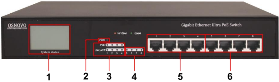
Рис. 3 Разъемы и индикаторы передней панели коммутатора SW-8080/THE
