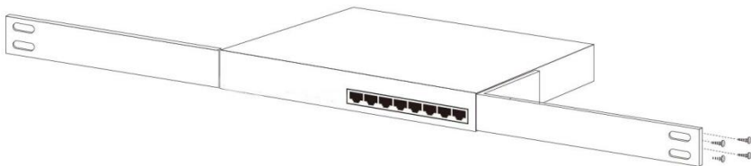
Рис. 9 Установка боковых креплений на коммутатор SW-8080/THE
