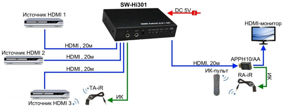
Рис. 3 Пример подключения устройства SW-Hi301
