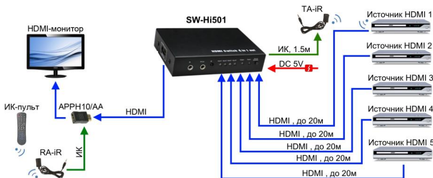
Рис. 4 Схема подключения SW-Hi501
