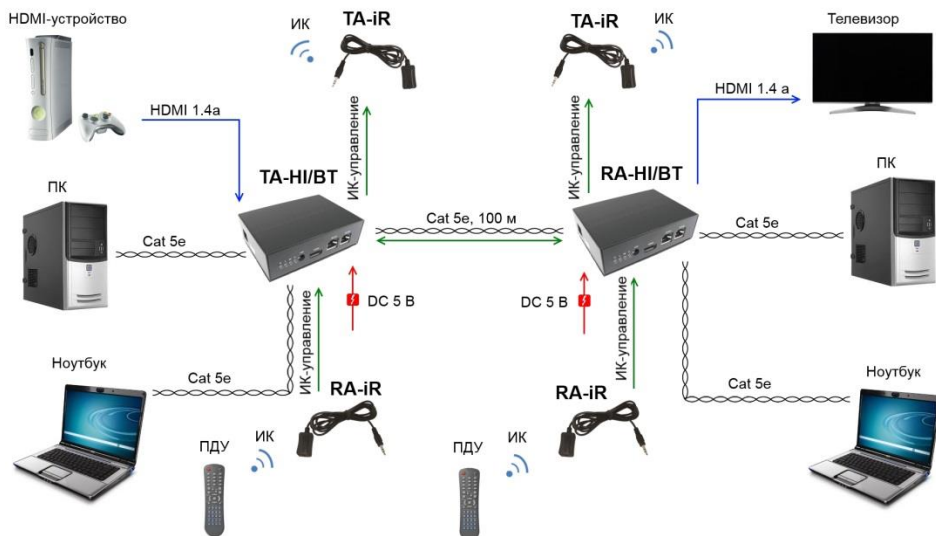
Рис. 3 Схема подключения TA-Hi/BT+RA-Hi/BT / TA-Hi/BT(W)+RA-Hi/BT(W)
