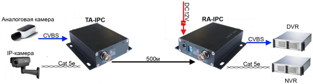
Рис.3 Схема подключения
