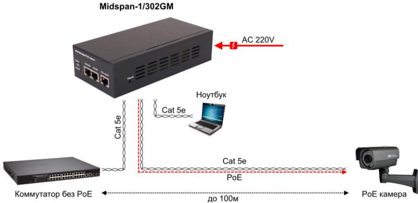
Рис.3 Типовая схема подключения уличного инжектора Midspan-1/302GM
