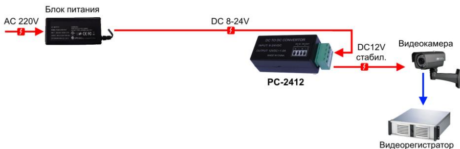
Рис.3 Схема подключения преобразователя PC-2412
