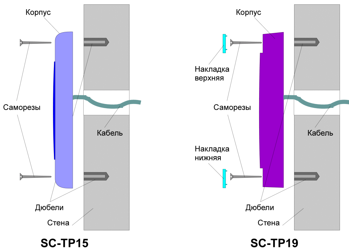
Рисунок 1. Крепление контроллеров.
