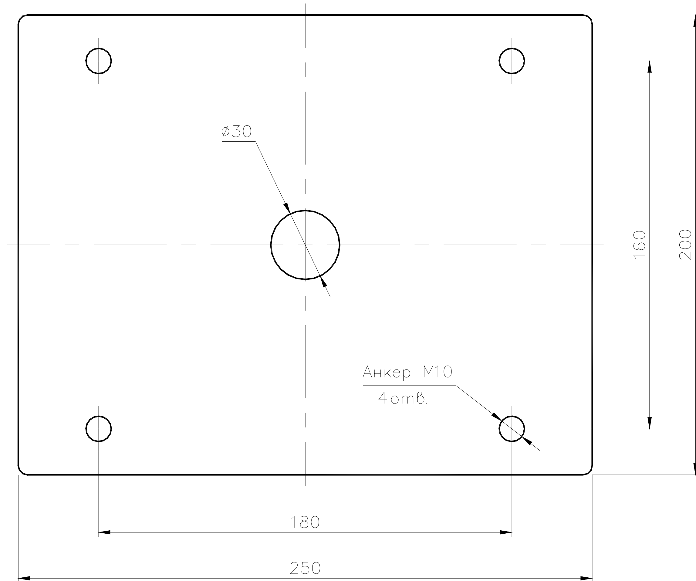
Рис. 12.3 Шаблон разметки основания стойки PW-500
