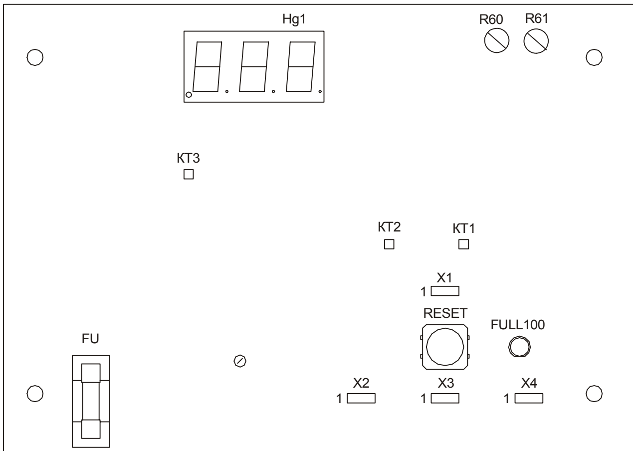
Рис. 12.1 Плата управления
