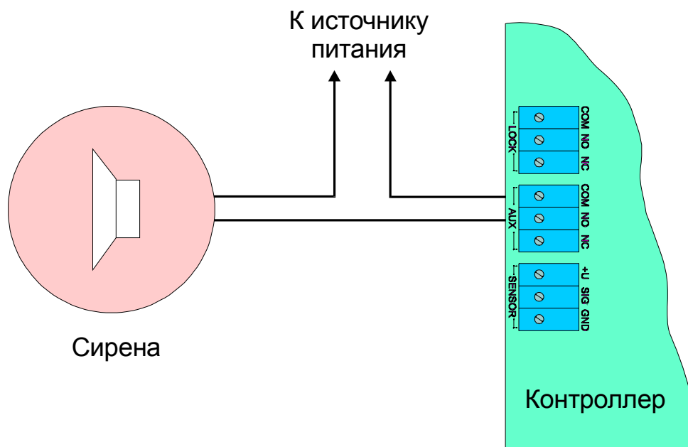
Рис. 11. Подключение к дополнительному реле
