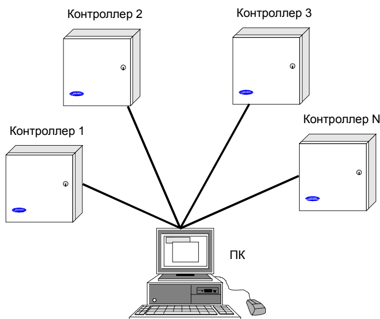
б). Соединение контроллеров по топологии «Звезда»
