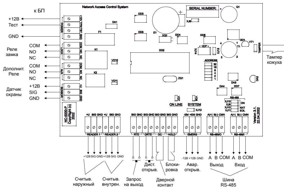
Рис. 2. Печатная плата контроллера NC-5000
