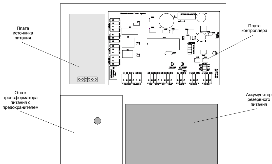
Рис. 1. Контроллер NC-5000
