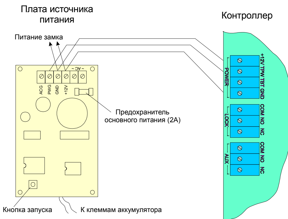
Рис. 15. Подключение источника питания к контроллеру
