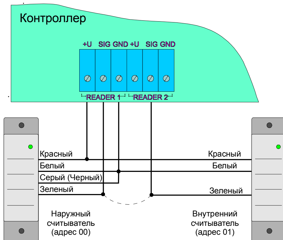
Рис. 4. Подключение считывателей серии NR-A0x к контроллеру NC-5000
