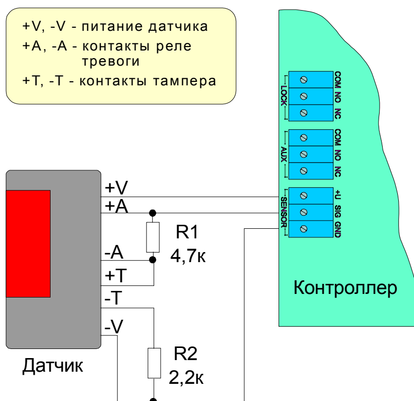
Рис. 10. Подключение охранного датчика
