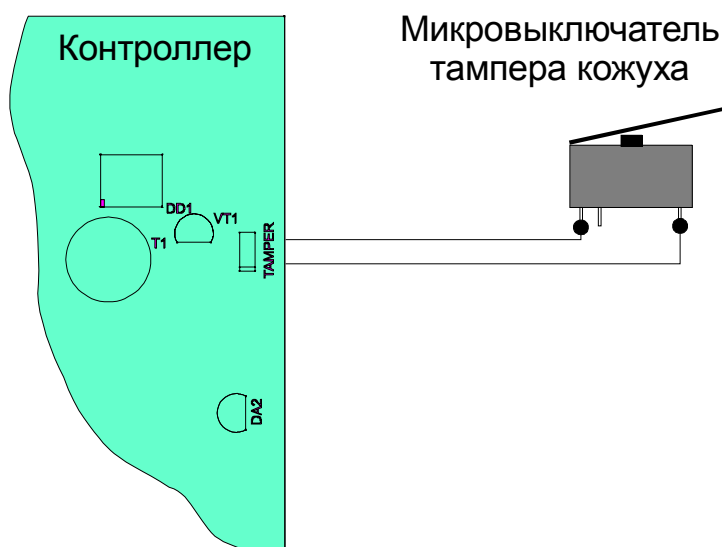
Рис. 12. Подключение тампера кожуха
