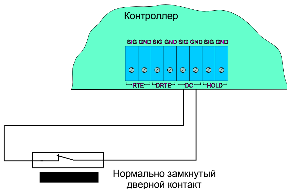
Рис. 6а. Подключение DC без контроля подводящих проводов
