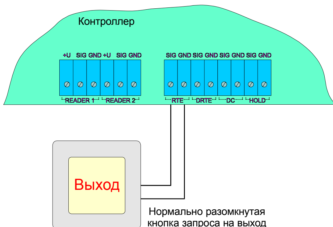
Рис. 5. Схема подключения кнопки запроса на выход
