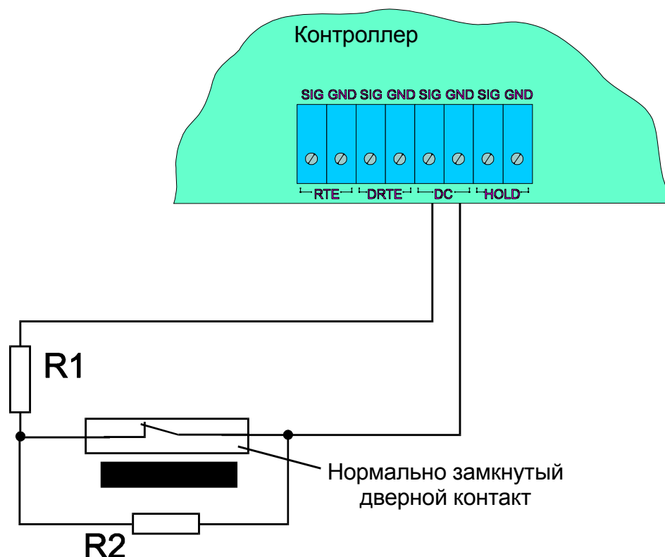
Рис. 6б. Подключение DC с контролем подводящих проводов
