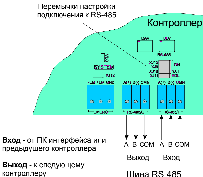
Рис. 17. Подключение контроллера к шине RS-485
