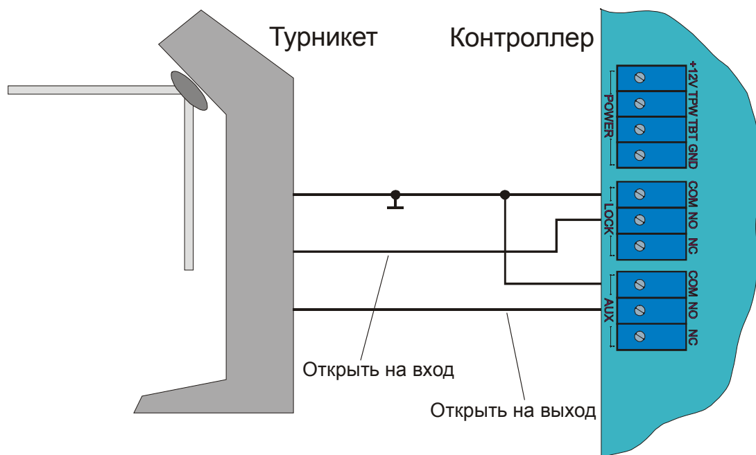
Рис. 9. Управление турникетом контроллерами версий NC5K06 и выше
