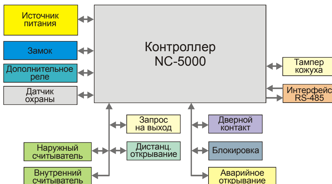
Рис. 3. Оборудование, подключаемое к контроллеру NC-5000
