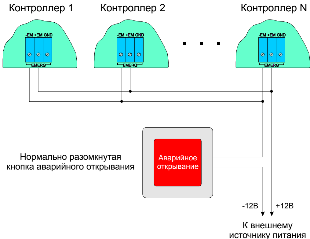
Рис. 14. Подключение одной кнопки к нескольким контроллерам
