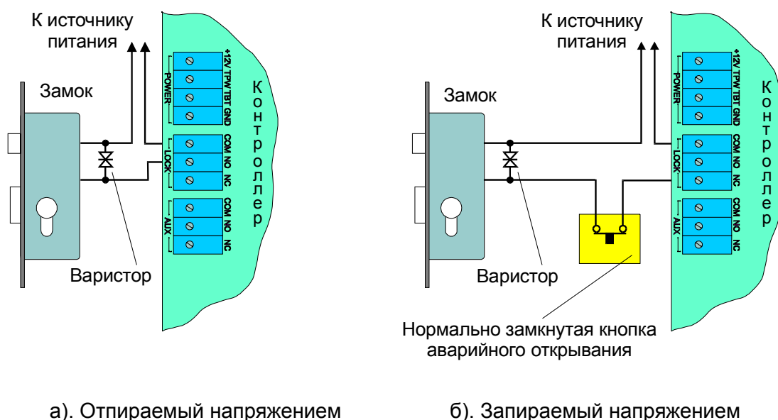
Рис. 7. Подключение замков к контроллеру
