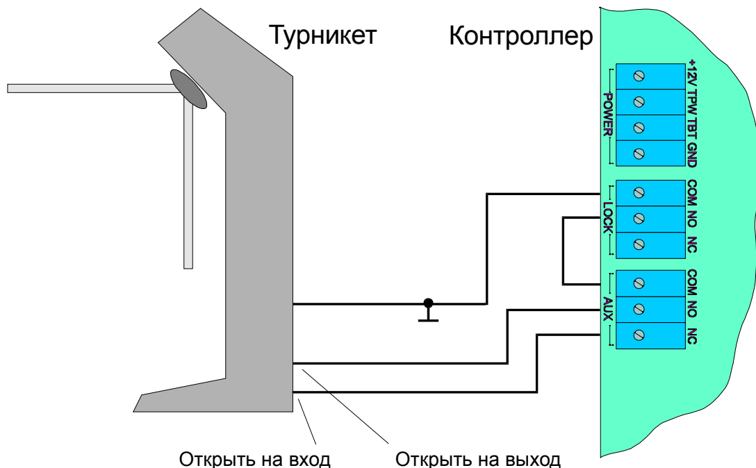
Рис. 8. Управление турникетом контроллерами NC-5000 ранних версий
