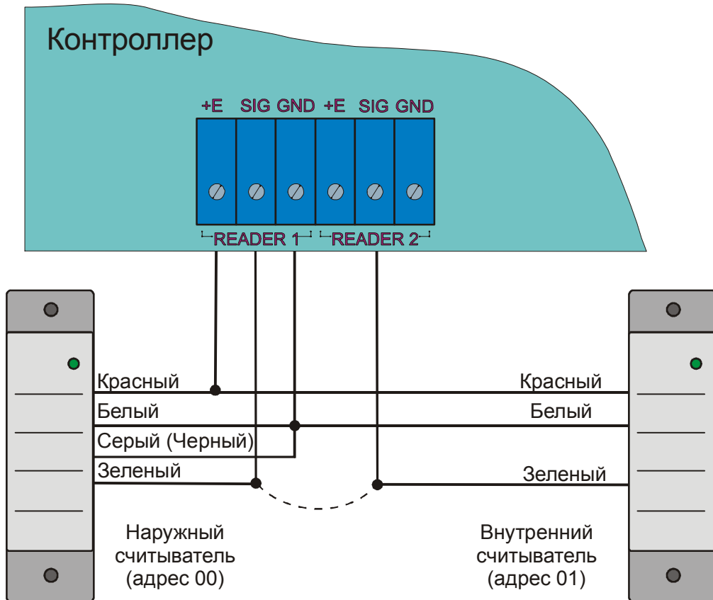
Рисунок 4. Подключение считывателей серии NR-A0x к контроллеру NC-32K.
