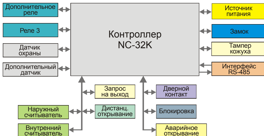
Рисунок 3. Оборудование, подключаемое к контроллеру NC-32K .
