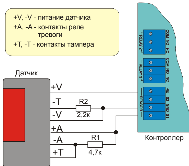
Рисунок 10а. Подключение охранного датчика.
