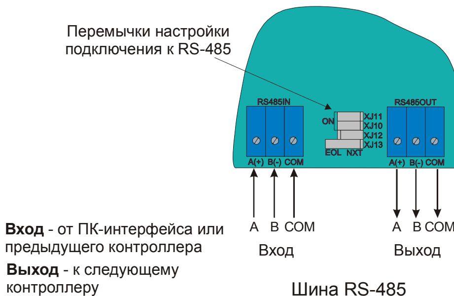
Рисунок 17. Подключение контроллера к шине RS-485.
