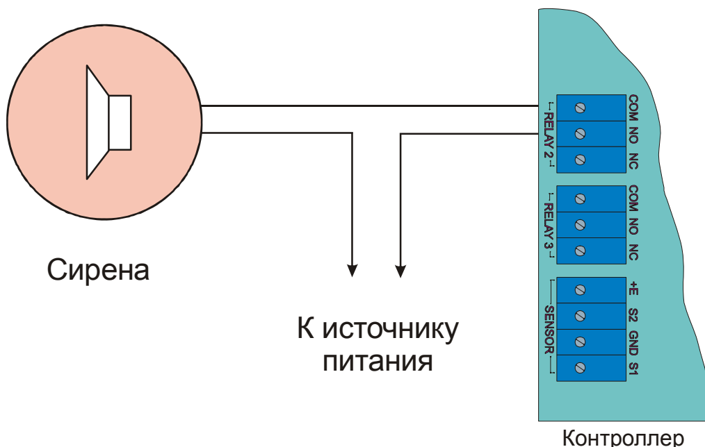
Рисунок 11. Подключение к дополнительному реле.
