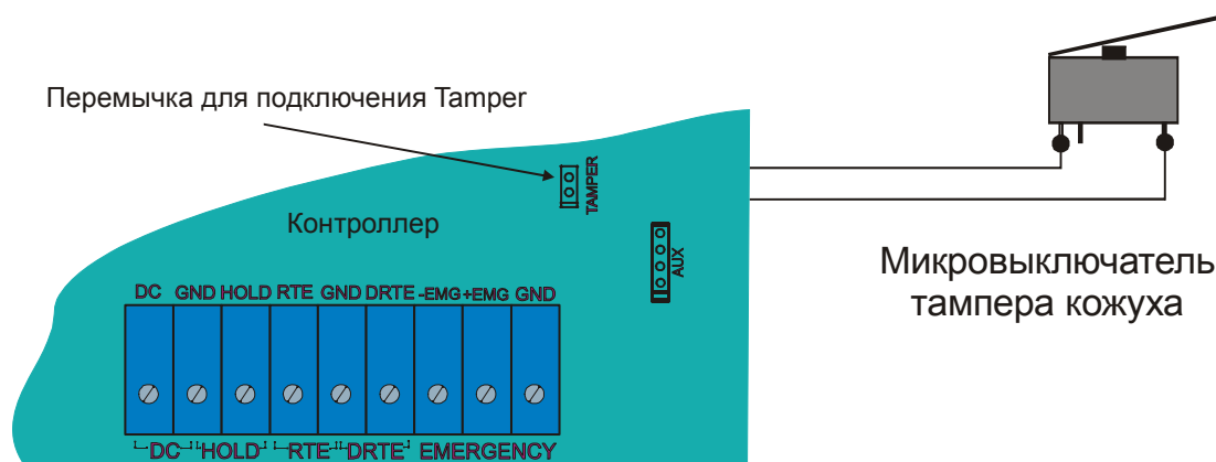
Рисунок 12. Подключение тампера кожуха.
