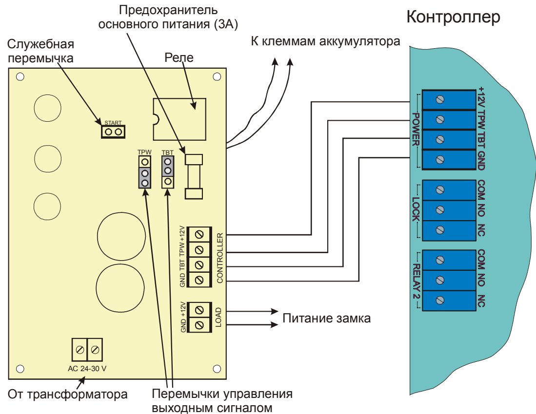
Рисунок 15. Подключение источника питания к контроллеру.
