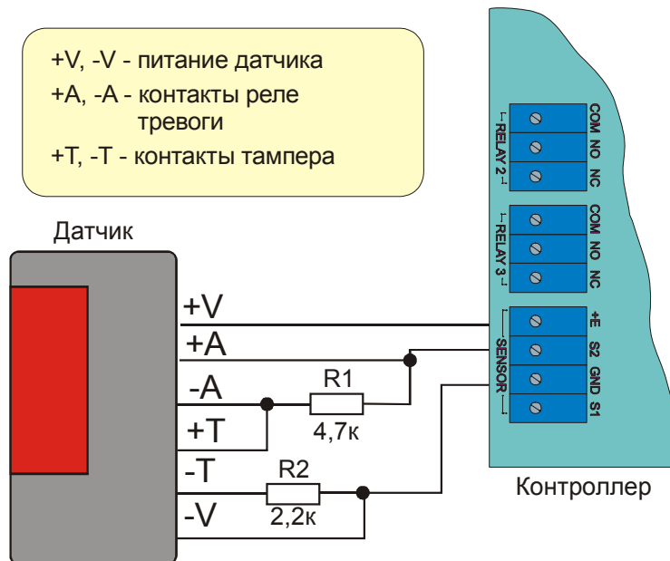
Рисунок 10б. Подключение дополнительного датчика.
