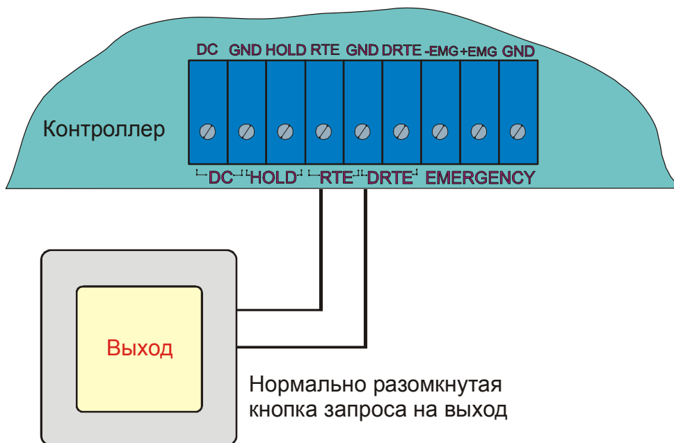
Рисунок 5. Схема подключения кнопки запроса на выход.
