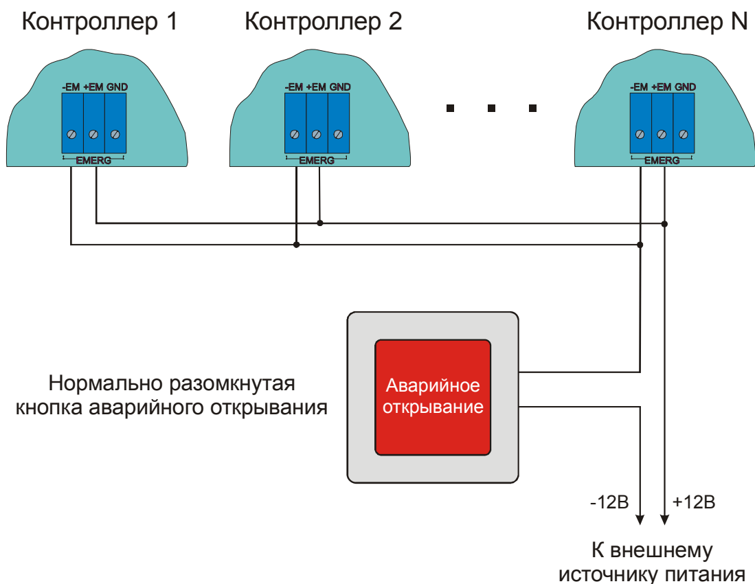
Рисунок 14. Подключение одной кнопки к нескольким контроллерам.
