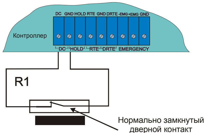
Рисунок 6. Подключение DC к контроллеру NC-32K .
