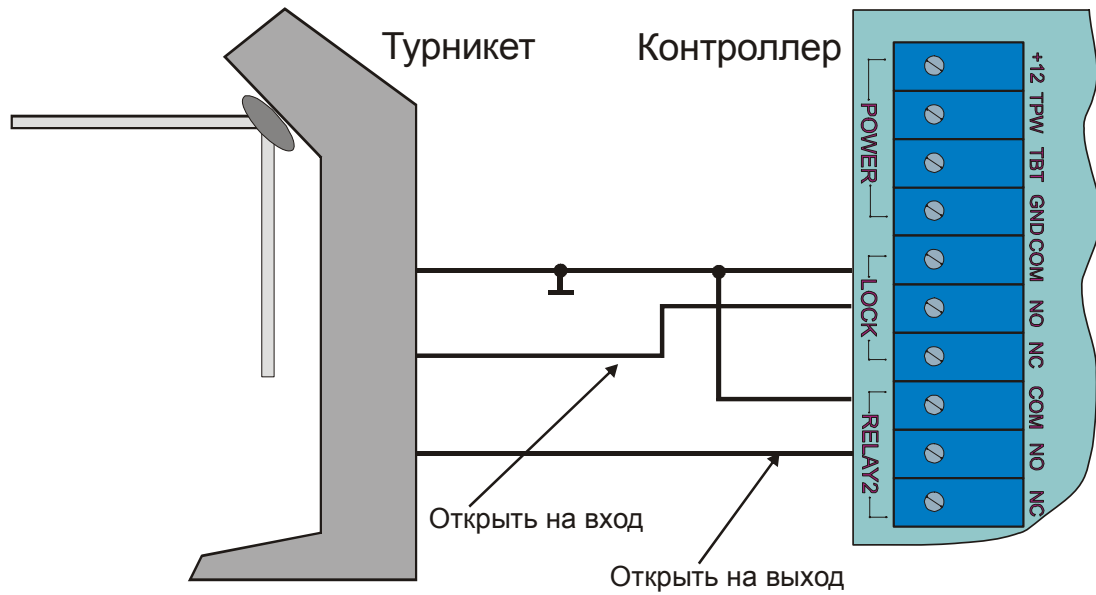
Рисунок 9. Управление турникетом контроллерами.
