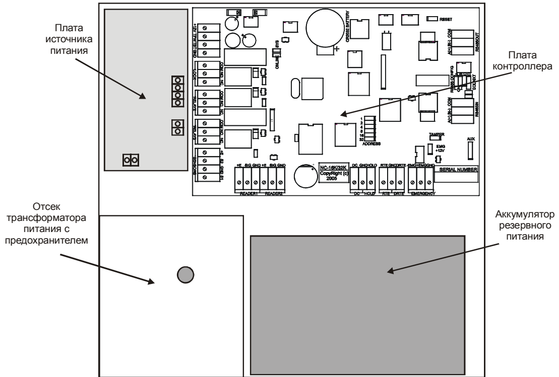
Рисунок 1. Контроллер NC-32K .
