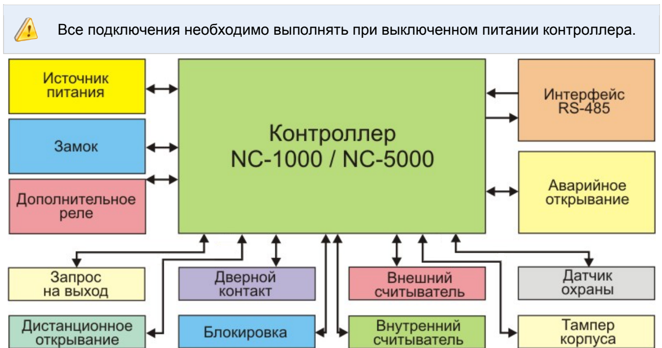
Рисунок 8. Оборудование, подключаемое к контроллерам NC-1000M / NC-5000
