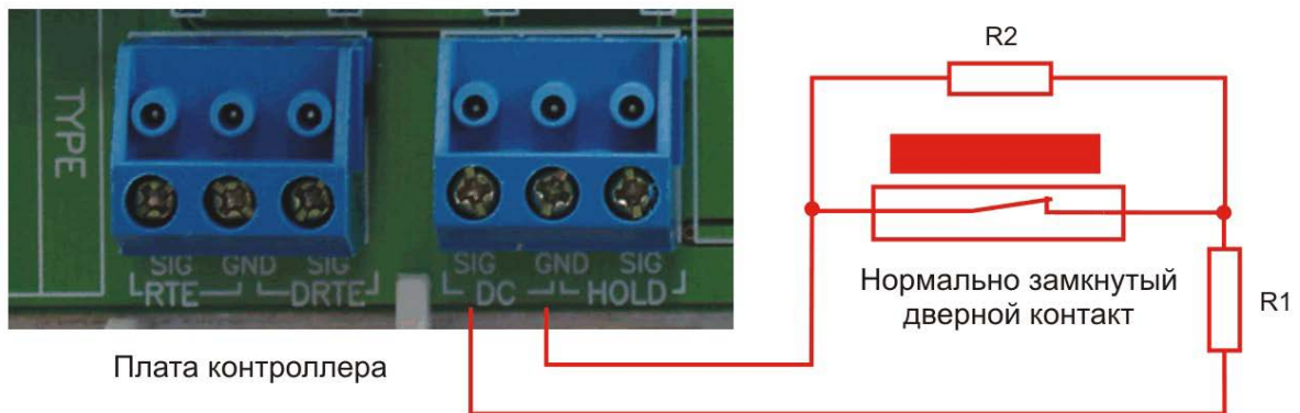
Рисунок 18. Подключение DC с контролем подводящих проводов
