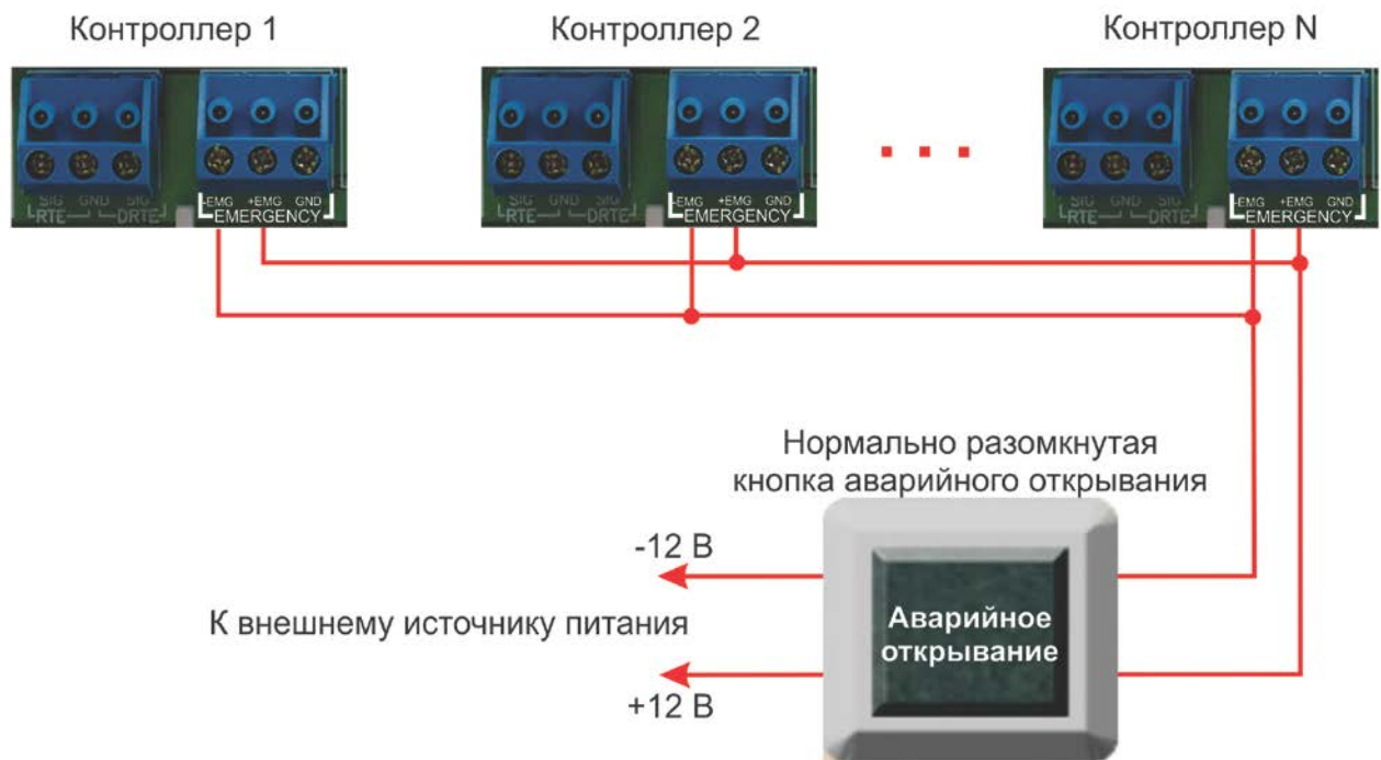
Рисунок 25. Подключение одной кнопки к нескольким контроллерам
