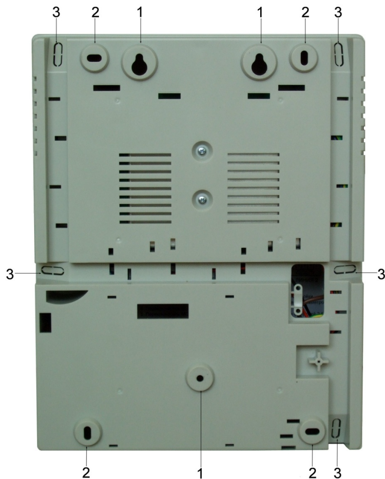
Рисунок 4. Монтажные отверстия
