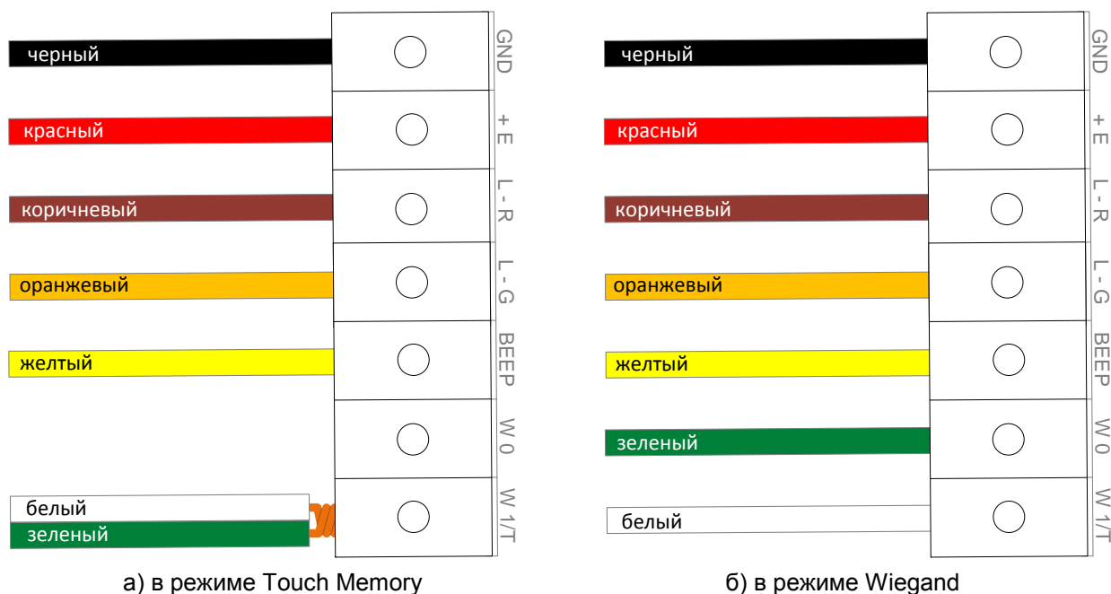
Рисунок 7. Подключение считывателя к интерфейсу NI-TW
