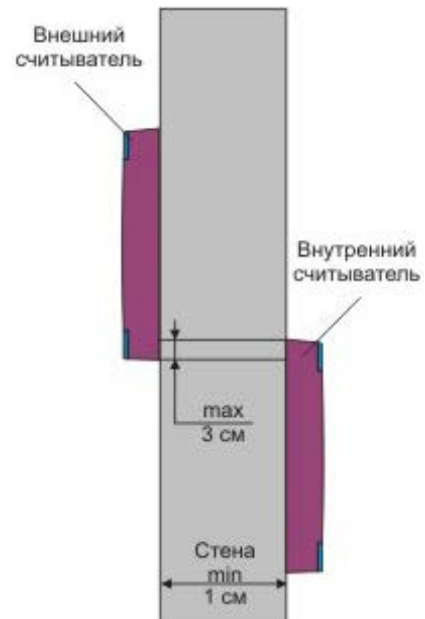
Рисунок 4. Крепление считывателей с разнесением по вертикали.
