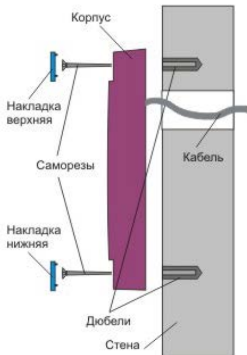
Рисунок 2. Крепление PR-EH16
