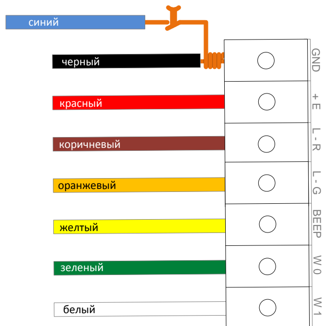
Рисунок 6. Пример подключения провода HOLD/SYNC для ручного включения режима блокировки
