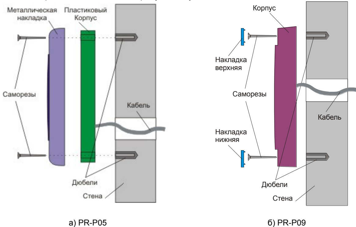
Рисунок 2. Крепление считывателей
