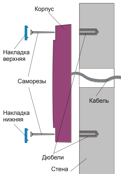
Рисунок 2. Крепление PR-P16
