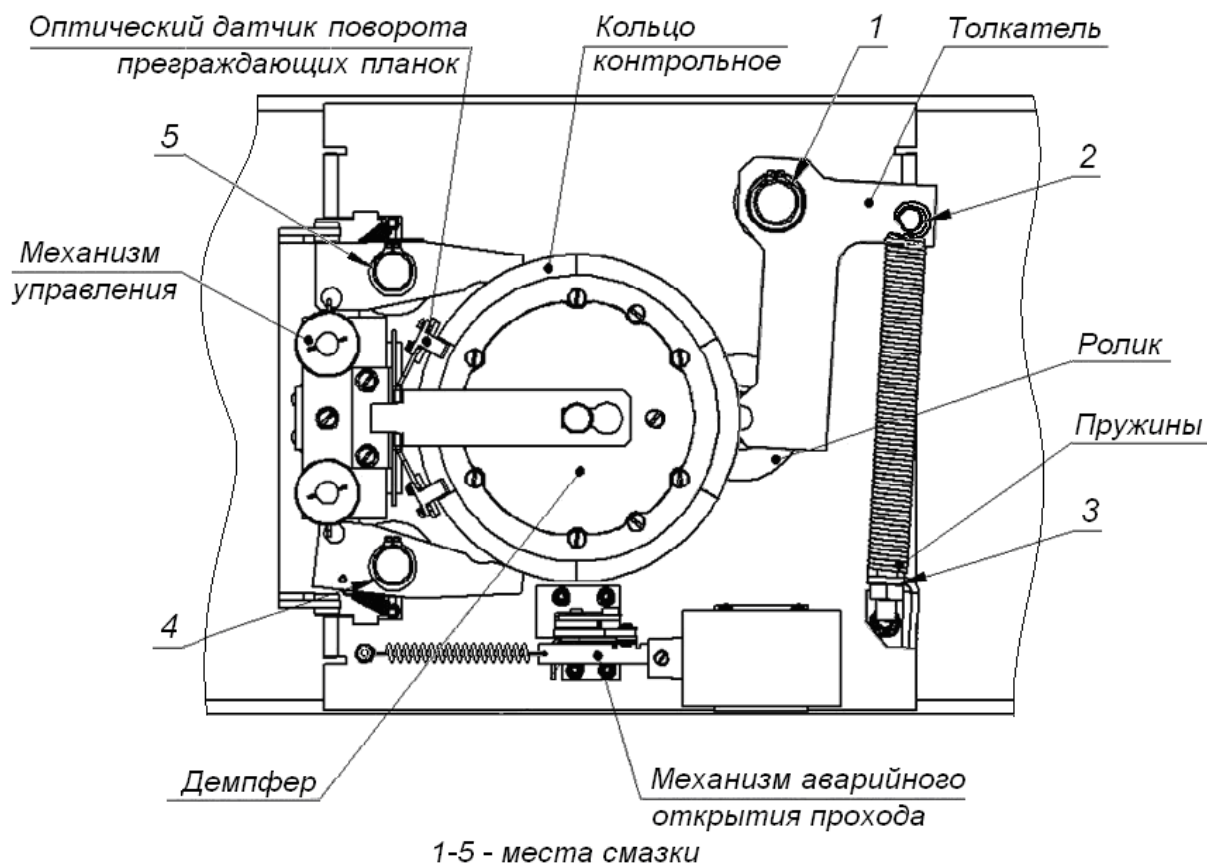
Рисунок 16. Узел вращения преграждающих планок турникета
