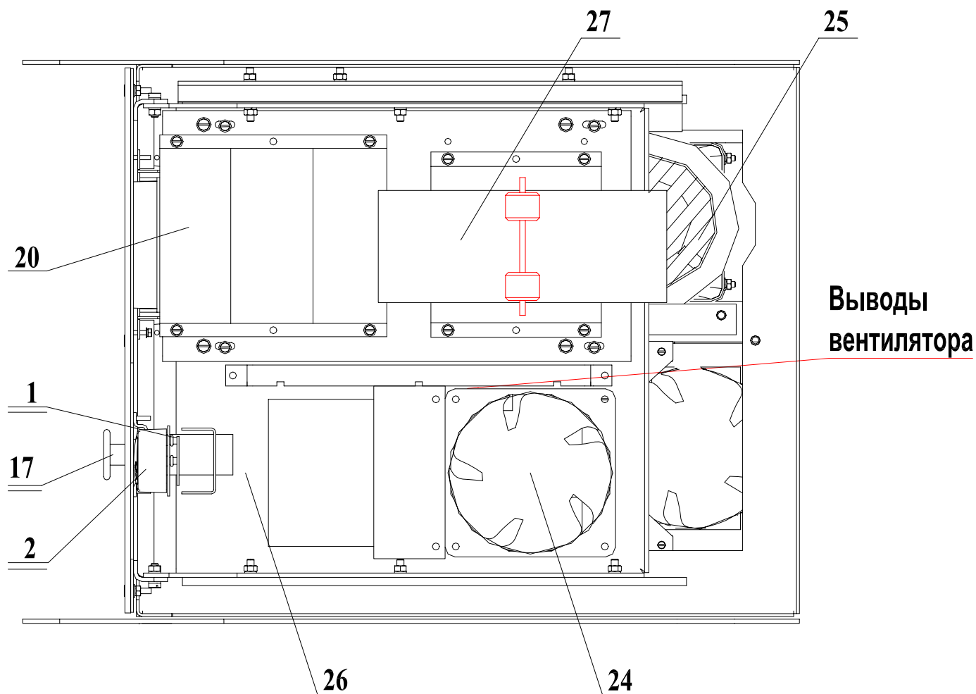
Рисунок 2 - Расположение аппаратуры в верхней части въездной стойки
