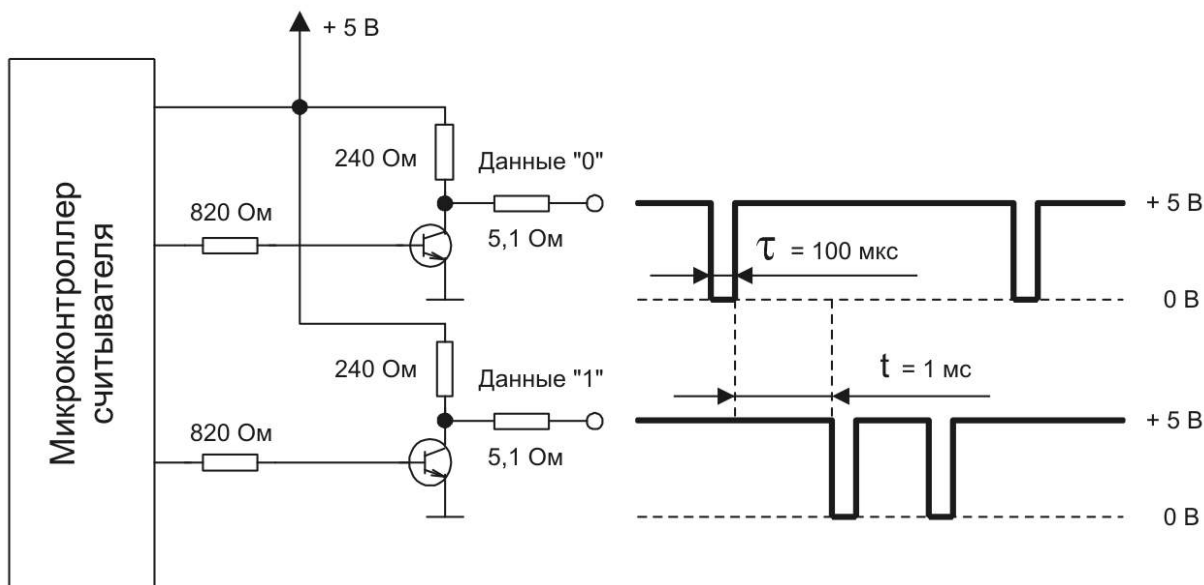
Рис.2. Схема формирования выходных сигналов считывателя и их эпюры.
