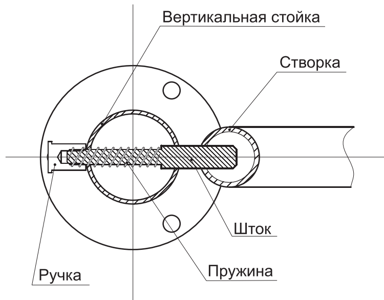
Рисунок 10 – Установка штока стопорного узла
