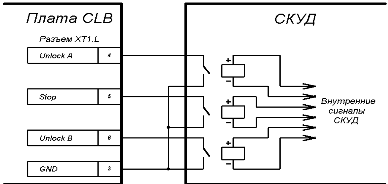
Рисунок 5 – Управляющий элемент СКУД – нормально разомкнутый контакт реле
